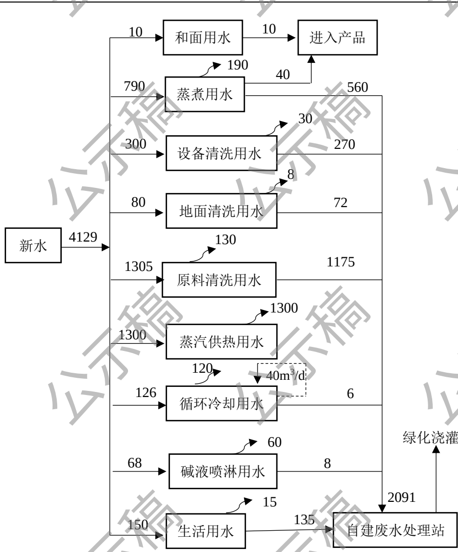
图 2-7 本扩建项目水平衡图 (单位: m³/a)
