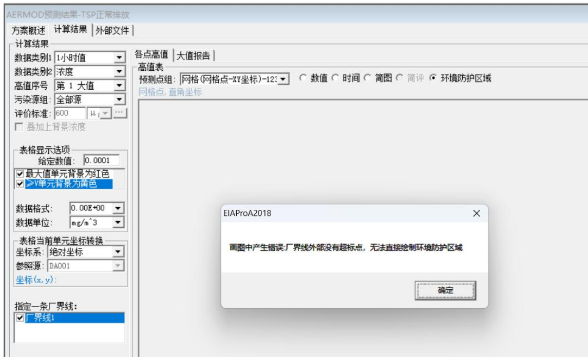
图 4-3 颗粒物正常排放预测结果
