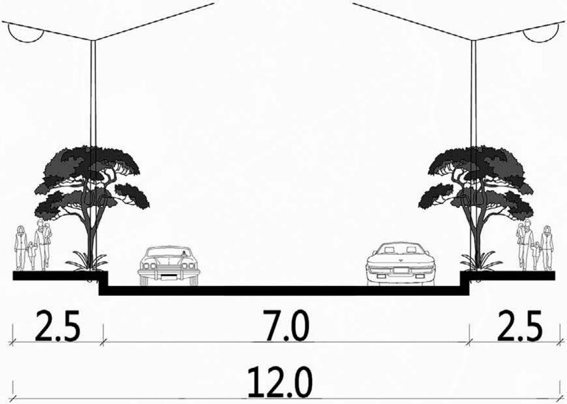
A-A 道路横断面
