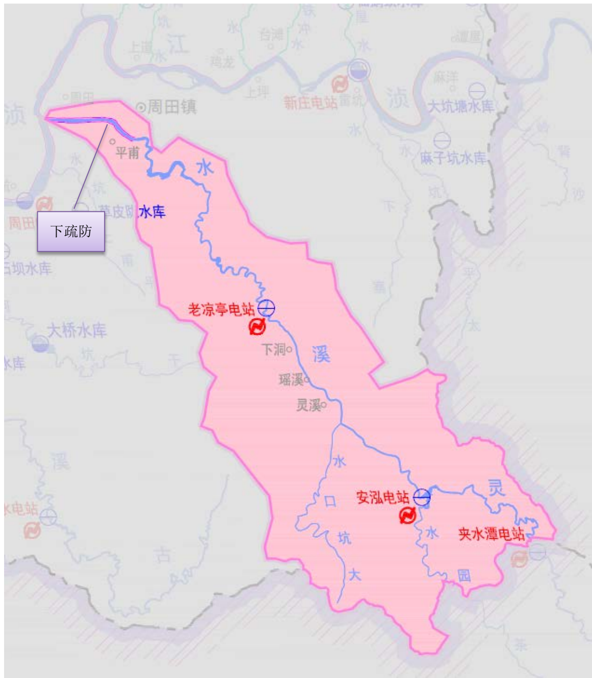
图 6-8 灵溪河流域防洪工程总体布局图
