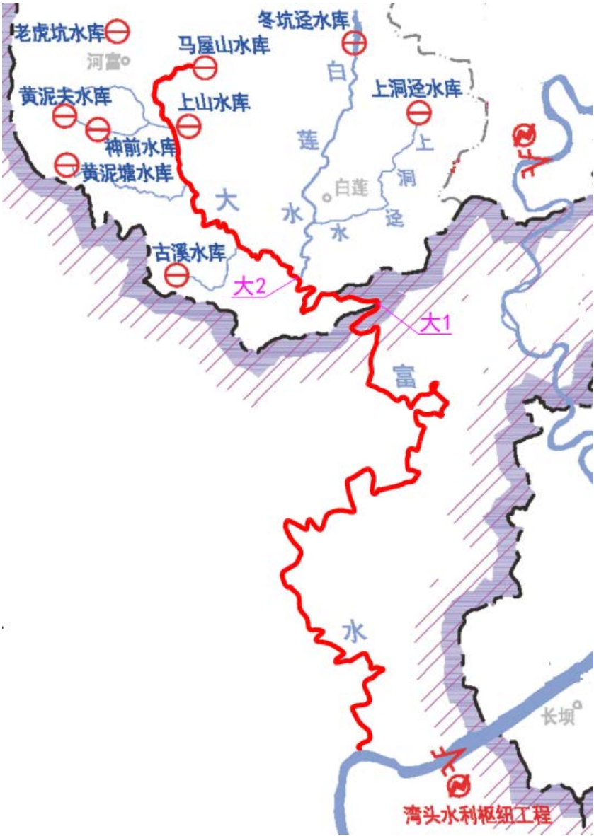
图 5-8 大富水文计算断面示意图
