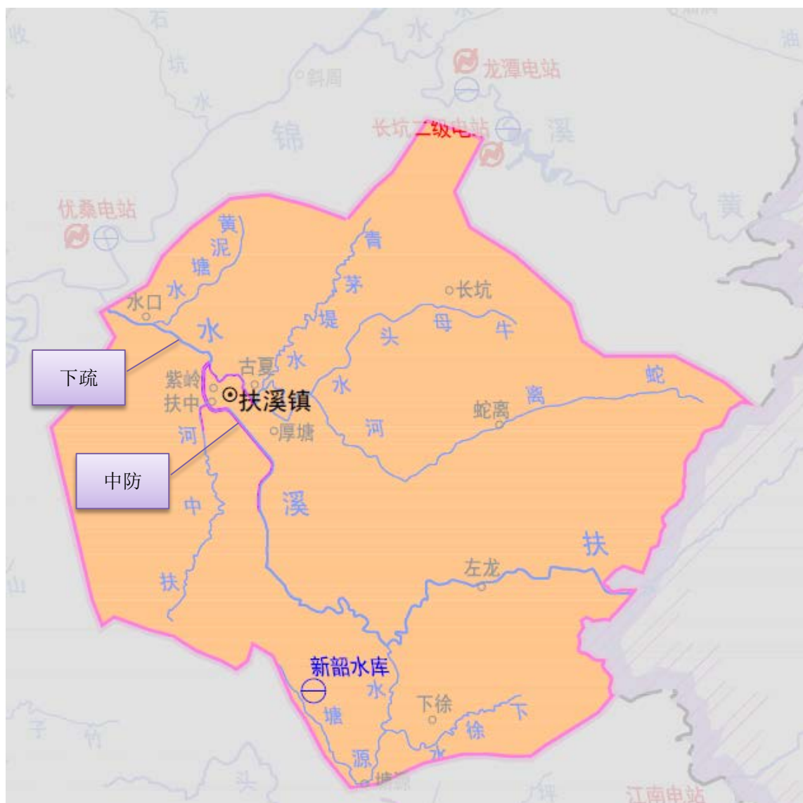
图 6-5 扶溪水流域防洪工程总体布局图
