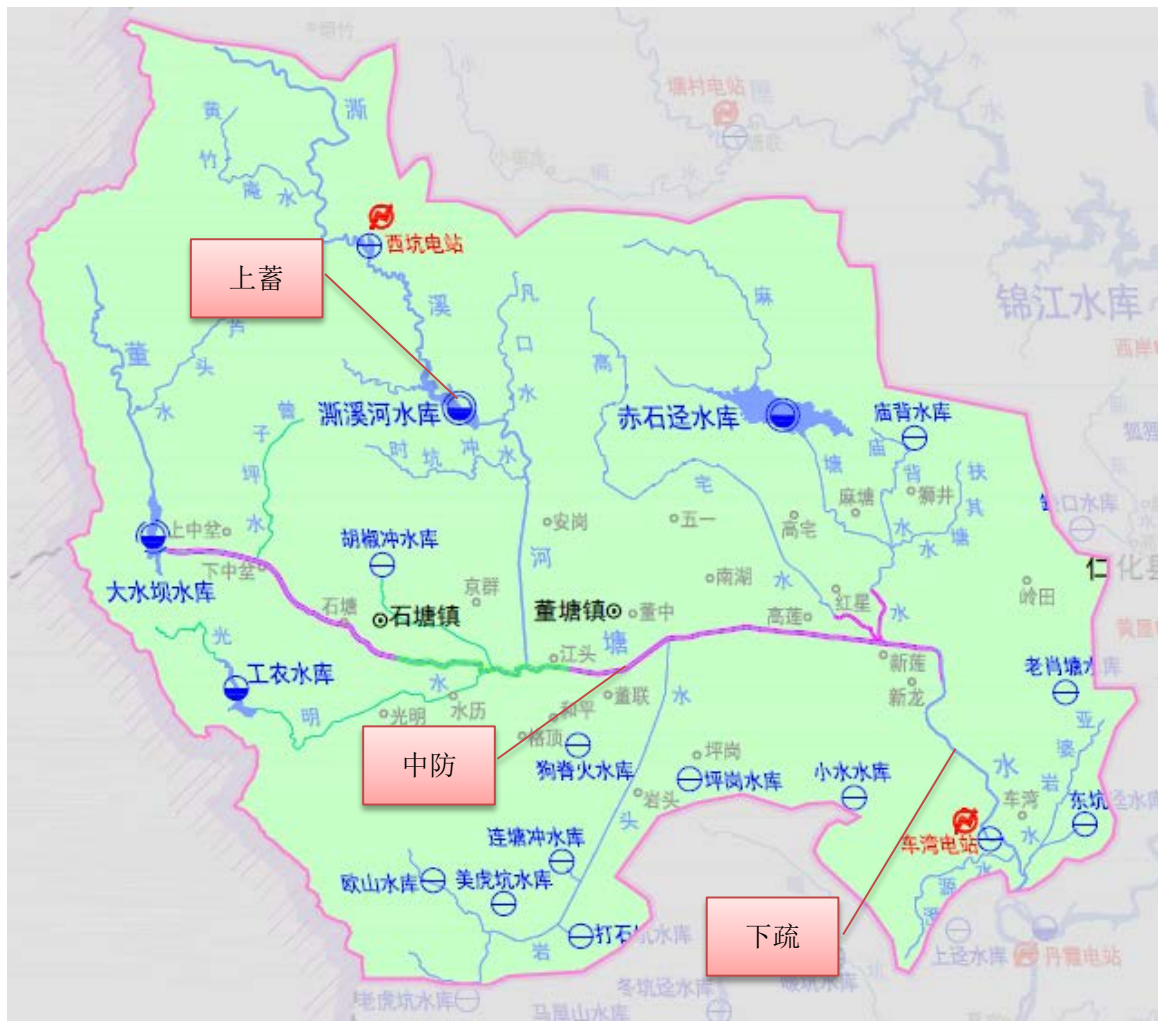
图 6-2 董塘水流域防洪工程总体布局图
