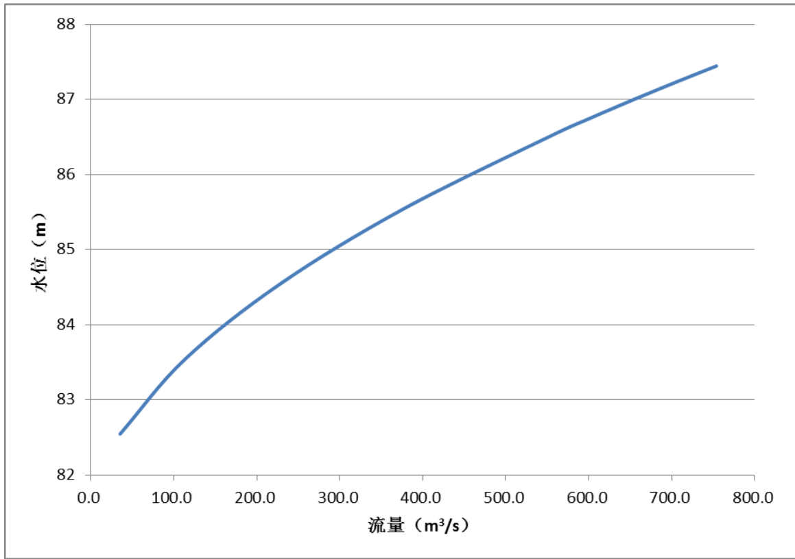
图 5-10 百顺水计算起始断面水位流量关系
