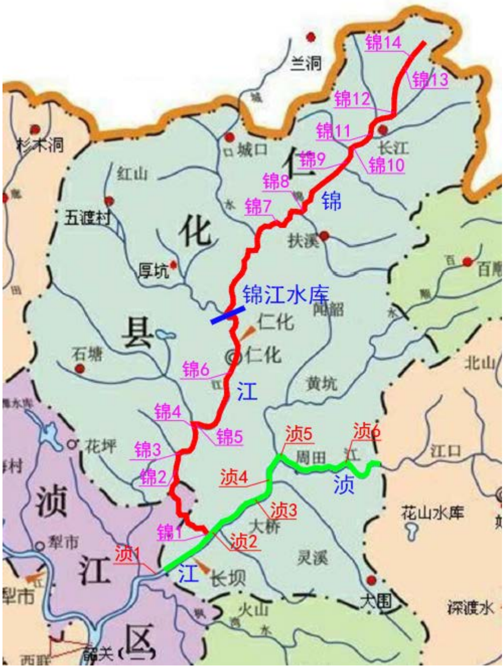
图 5-2 贞江、锦江水文计算断面示意图
