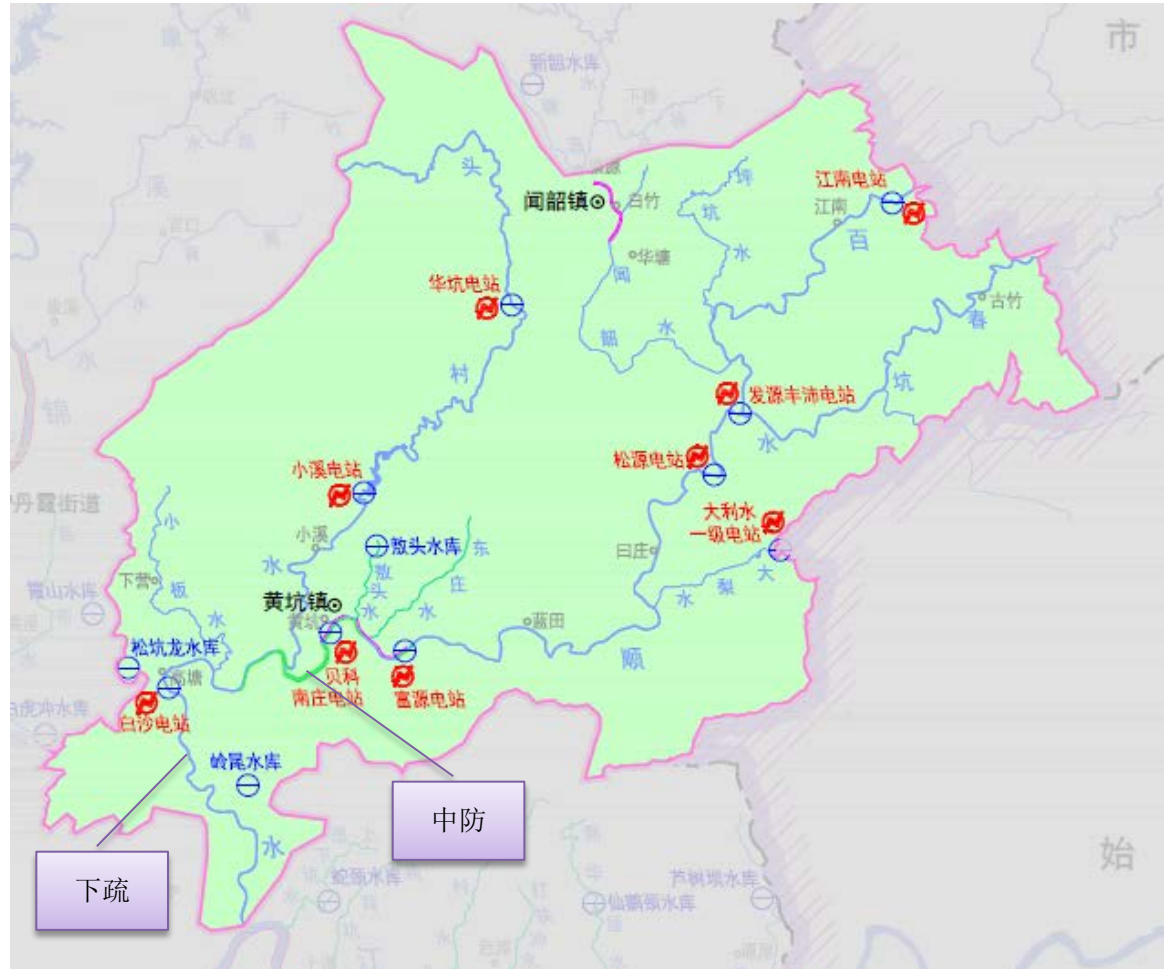
图 6-6 百顺水流域防洪工程总体布局图
