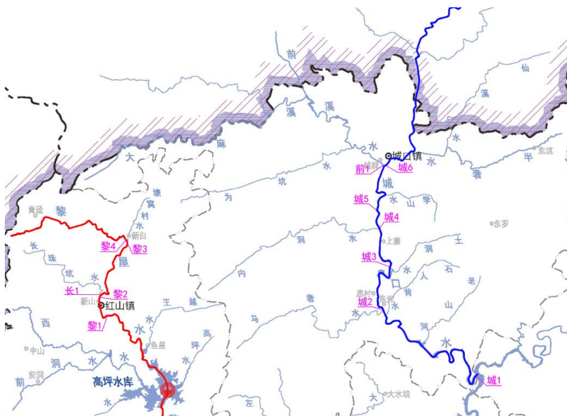
图 5-4 黎屋水、城口水水文计算断面示意图
