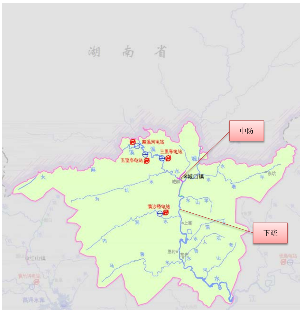
图 6-4 城口水流域防洪工程总体布局图
