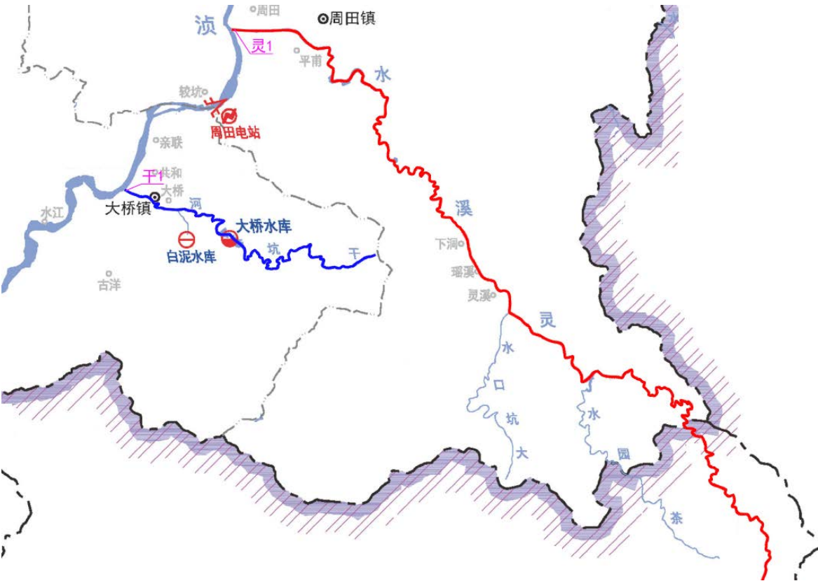
图 5-7 灵溪水、干坑河水文计算断面示意图
