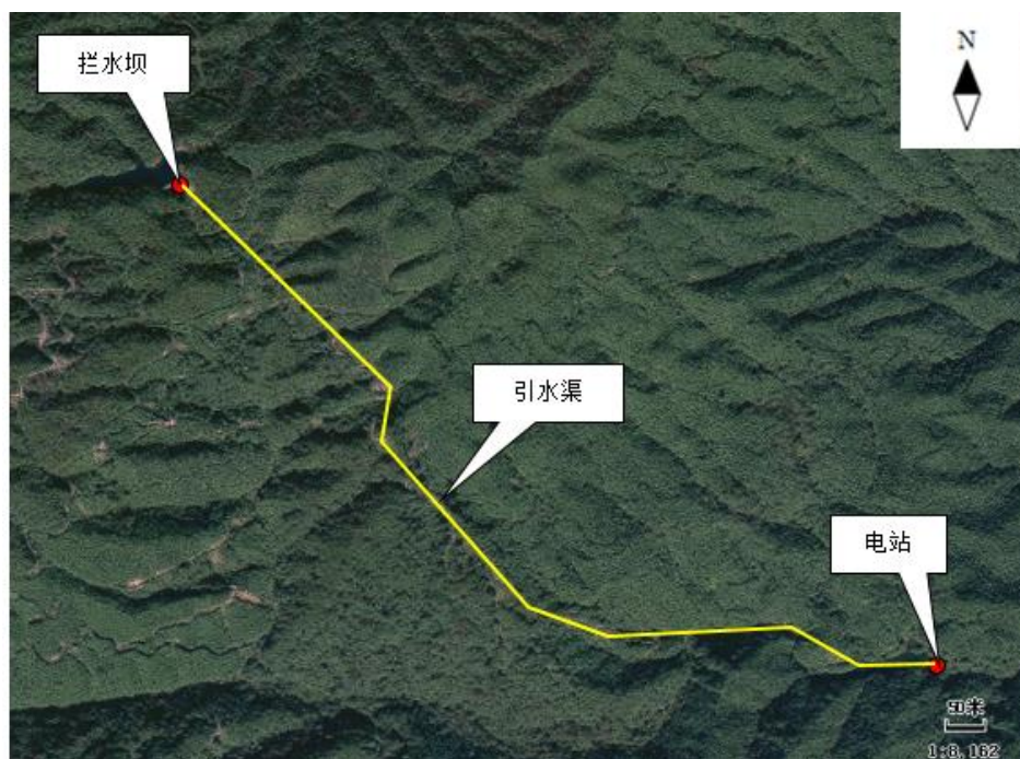
图 2-3 项目总体布置图
