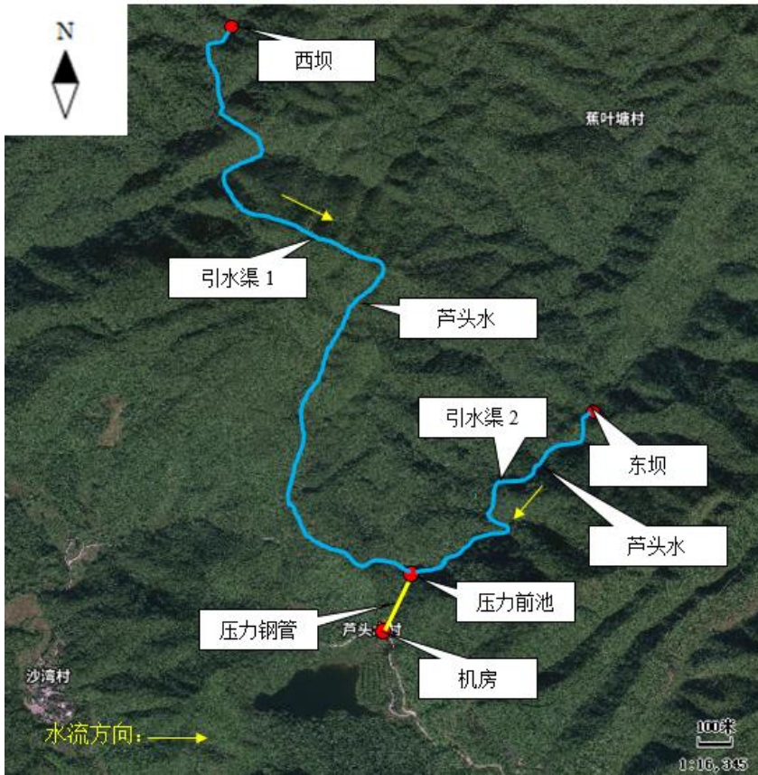
图 2-3 项目总体布置图
