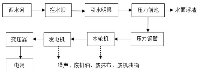
图 2-5 工程运行方式图
