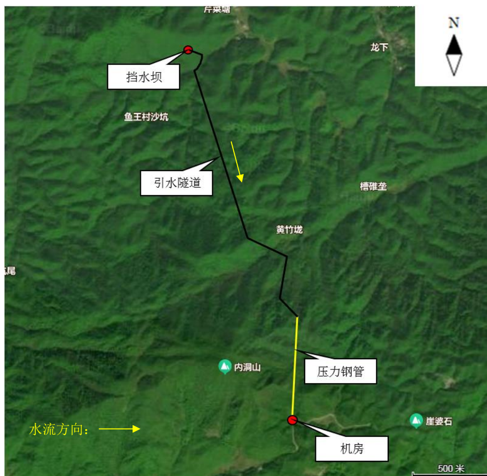
图 2-3 项目总体布置图
