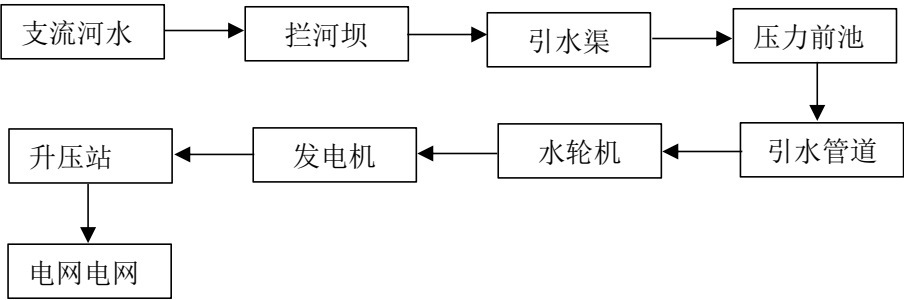
图 2-1 工程运行方式图
