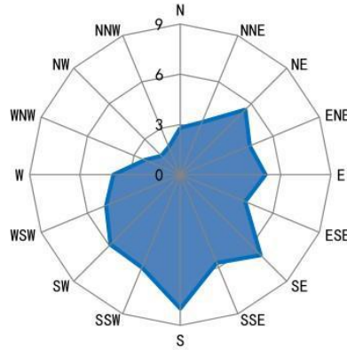
图 6-1 仁化县近 20 年风向玫瑰图
