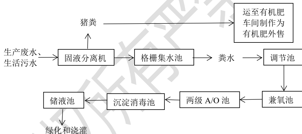
图 3-9 废水处理工艺流程图
