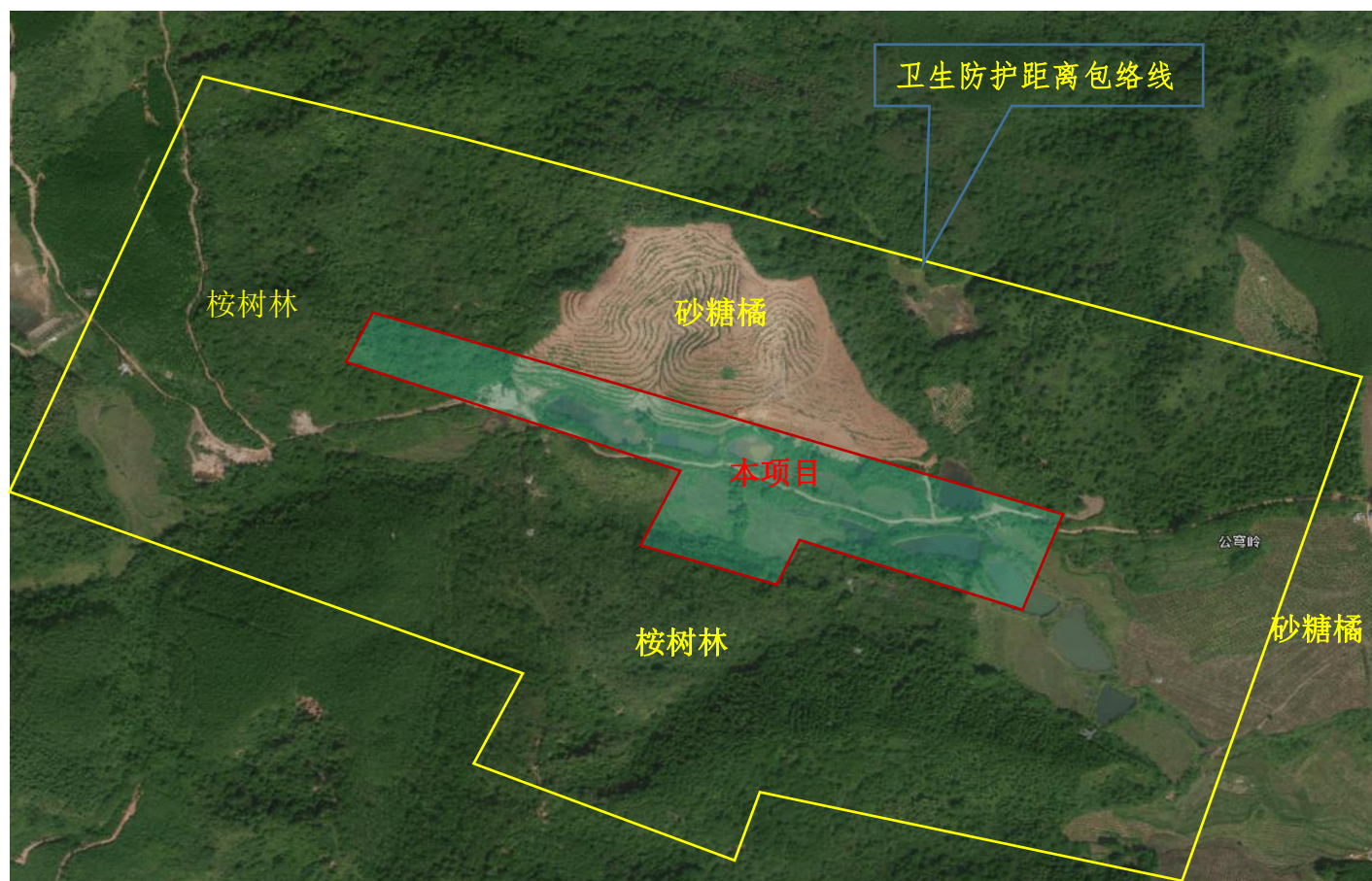
图 6-3 卫生防护距离包络线图
