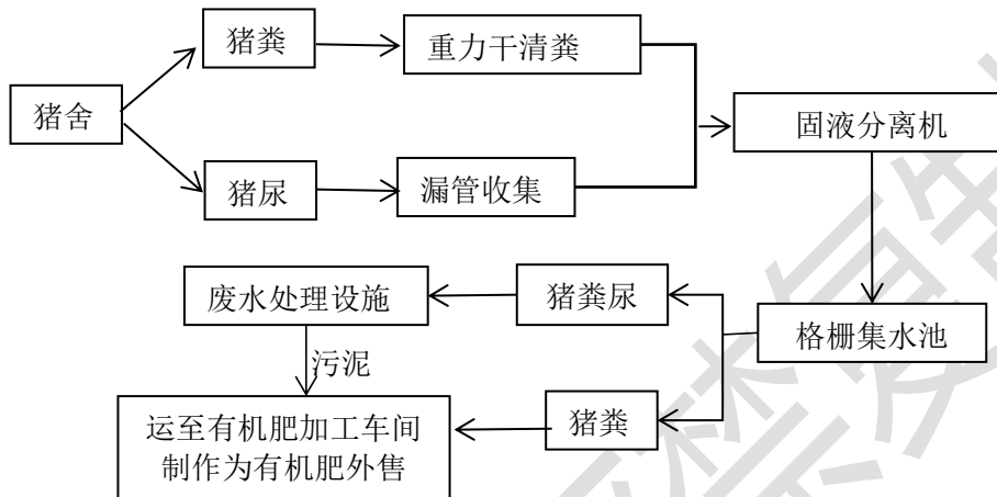
图 3-4 清粪及粪污处理工艺流程图
