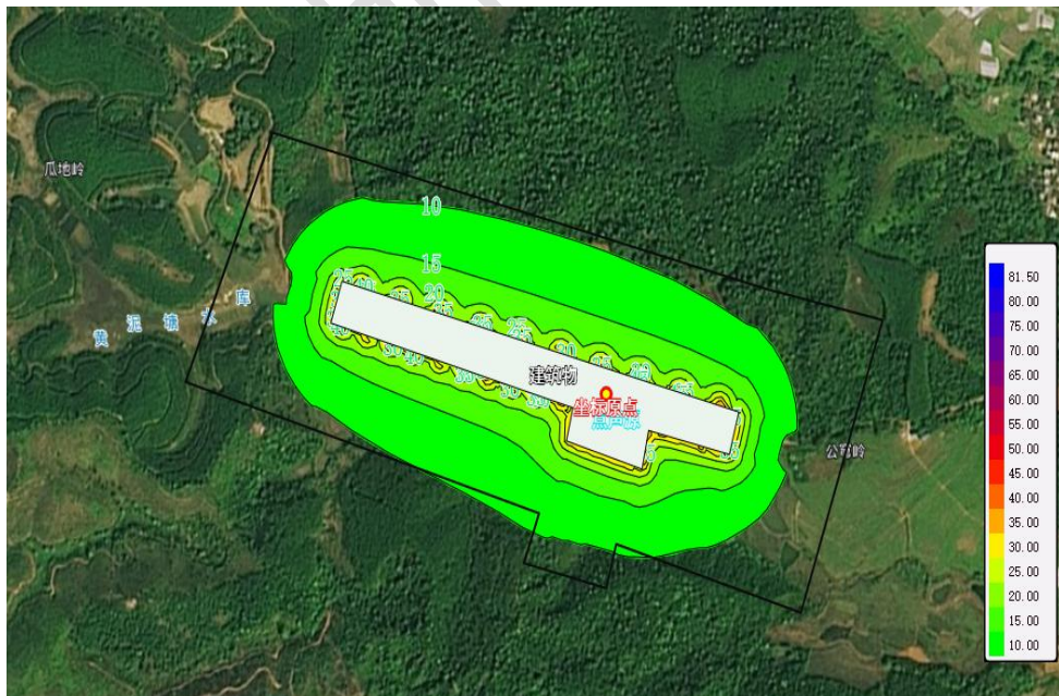
图 6-6 项目夜间噪声贡献值等值线图（单位：dB（A））
